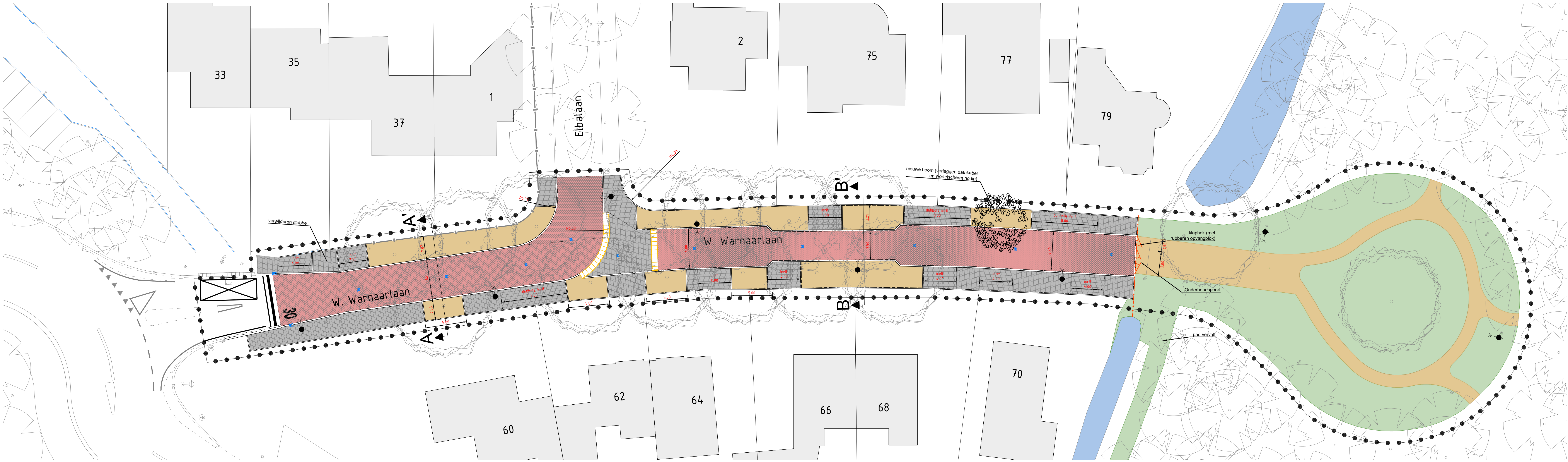
OVERZICHTSTEKENING SCHAAAL 1:200
